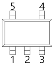
SOT-23-5L
